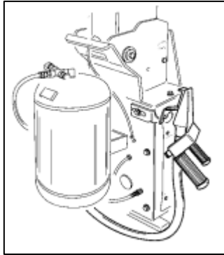
Schlauchloses Füllsystem
